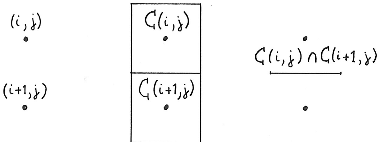
FIGURE 1. C(i, j) \cap C(i+1, j) \neq \emptyset .
